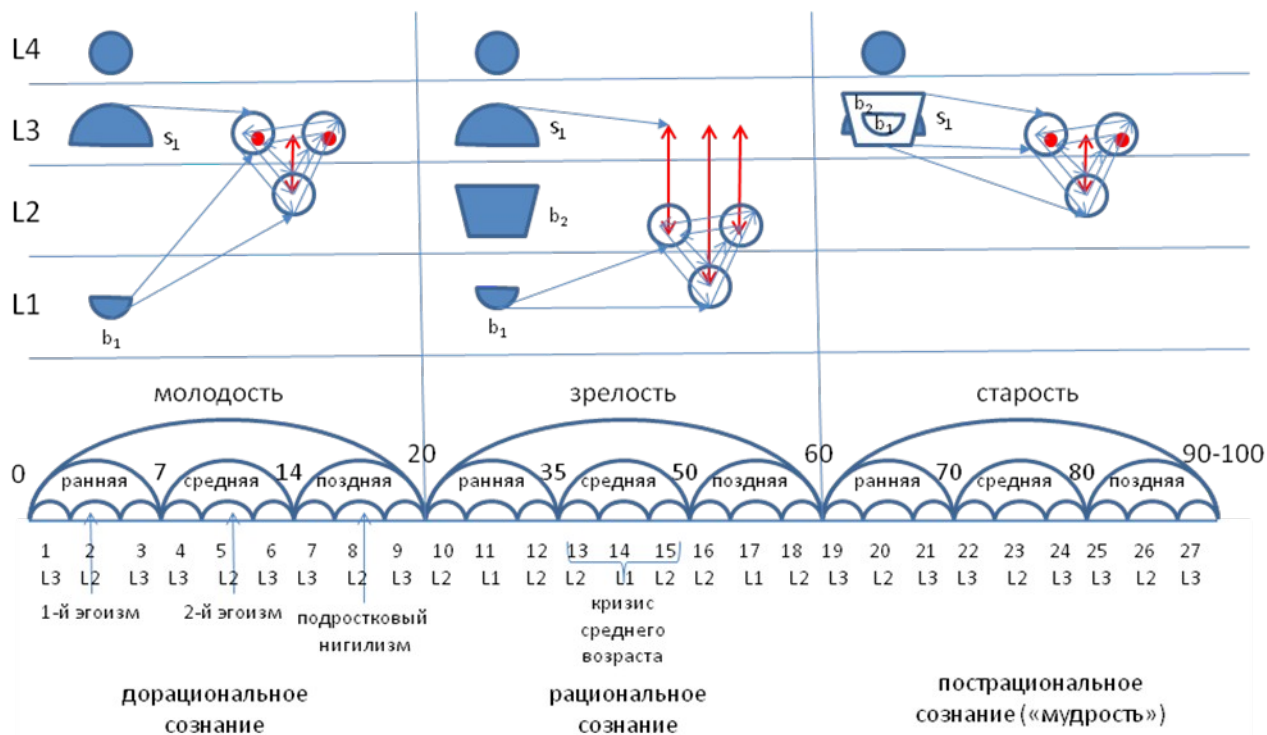
Рис.7. Представление жизненного цикла человека (от рождения до смерти) как спиральной модели развития в рамках Онтологии Мир-1.
