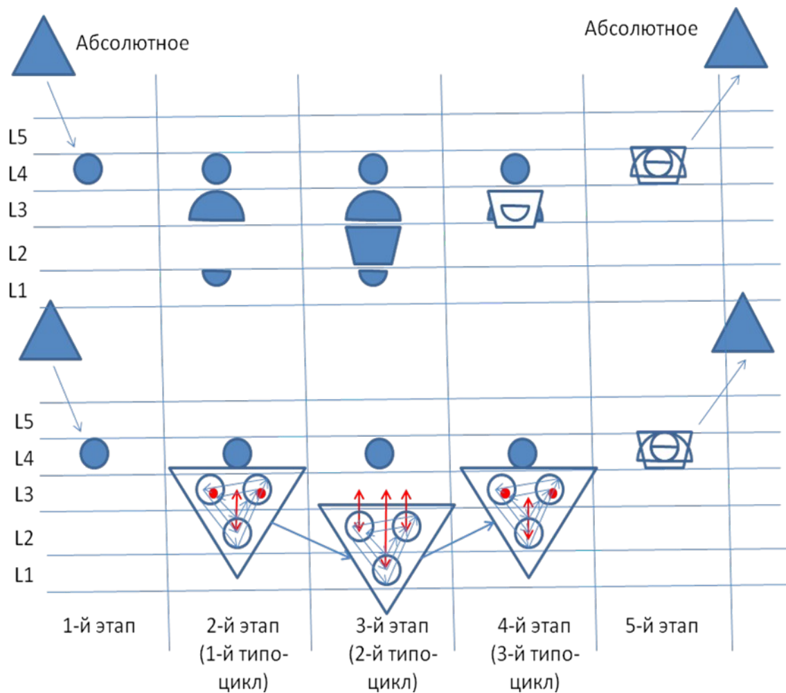
Рис.6. Координация внутренней (вверху) и внешней (внизу) моделей эпителиального развития для p=2 .
