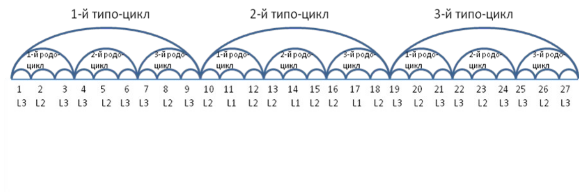
Рис.5. Структура 3-плерона воплощения третьего порядка в Онтологии Мир-1.
