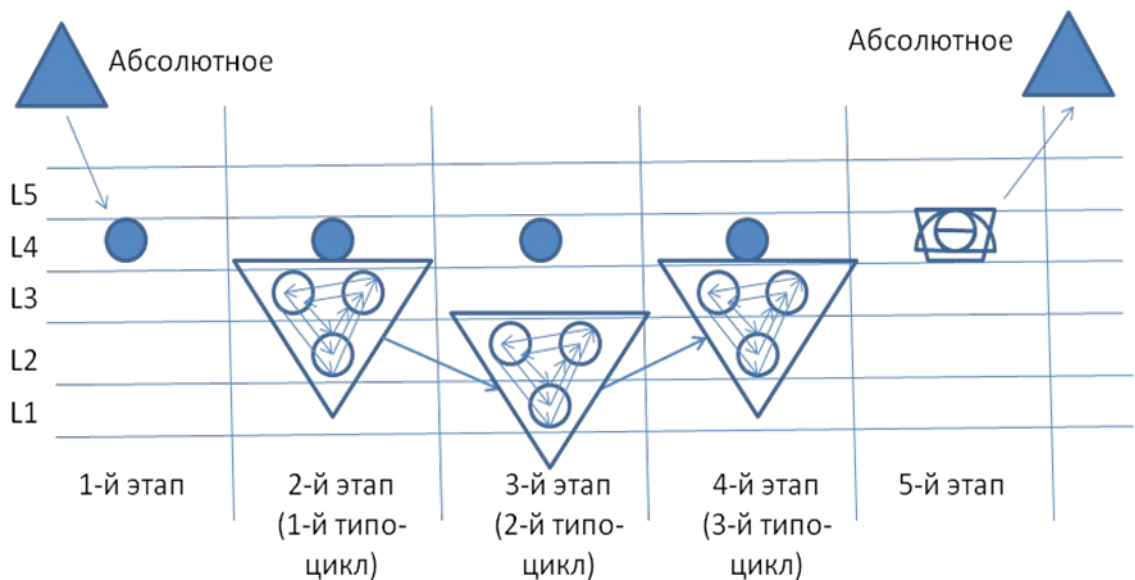
Рис.4. Представлен 3-плерон третьего порядка для модели внешнего развития эпителичности с типом-числом p=2 . Каждый тип-цикл изображен в виде прозрачного треугольника. В каждом треугольном контуре тонкими стрелками показано три родо-цикла. Каждый родо-цикл включает три прозрачных кружка как три видо-цикла. Три треугольных контура, расположенные в 1-3 тип-циклах, представляют весь плерон воплощения.
